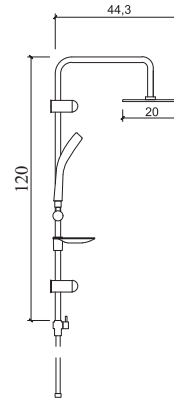
Cosmo Yağmur Duş Sistemi
