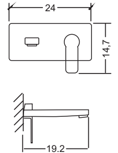
Ankastre Krom / Siyah Lavabo Armatürü
