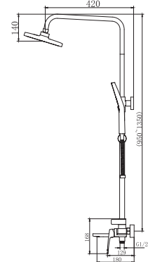
Zeno Krom / Gun Metal Duş Sistemi
