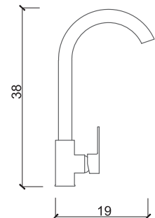
Kuşu Eviye Armatürü
