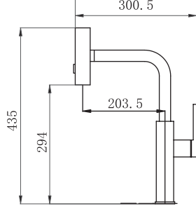
Inox Lotus Smart Spiralli Eviye Armatürü
