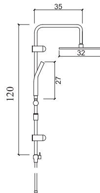
Nardo Yağmur Duş Sistemi
